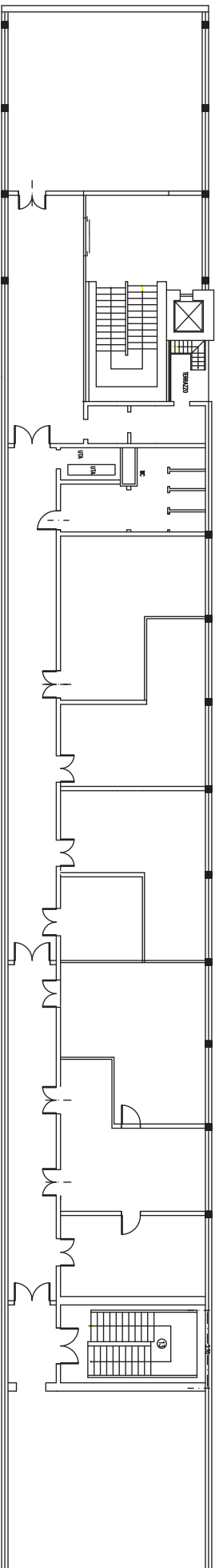
PIANTA PIANO TERZO - STATO DI PROGETTO
